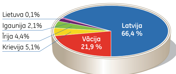
Ģeogrāfiskais sadalījums
